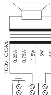
Leistungsanschlussbelegung
