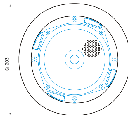
Frontansicht mit Gitter entfernt
